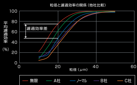
【粒径と濾過効率の関係 グラフ】 上のグラフはスラッジ(異物)の粒径と濾過効率の関係を示したグラフです。濾過効率がノーマル比で最大36%向上している事が認められます。
