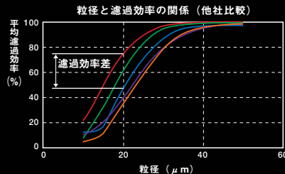
グラフは、スラッジ(異物)の粒径と濾過効率の関係を示したもので、濾過効率がノーマル比で最大36%向上していることが認められます。
