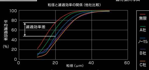
【粒径と濾過効率の関係 グラフ】
