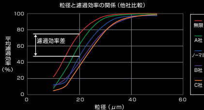
【粒径と濾過効率の関係グラフ】 上のグラフはスラッジ(異物)の粒径と濾過効率の関係を示したグラフです。濾過効率がノーマル比で最大10%向上している事が認められます。
