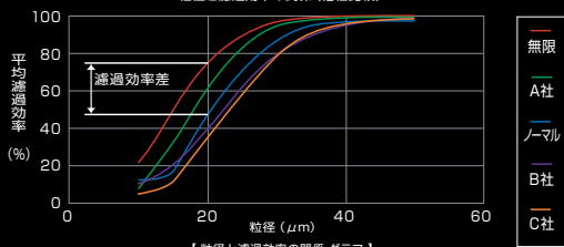
【粒径と濾過効率の関係 グラフ】 上のグラフはスラッジ（異物）の粒径と濾過効率の関係を示したグラフです。 濾過効率がノーマル比で最大38%向上している事が認められます。
