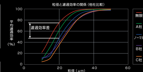
【粒径と濾過効率の関係グラフ】上のグラフはスラッジ(異物)の粒径と濾過効率の関係を示したグラフです。濾過効率がノーマル比で最大36%向上している事が認められます。
