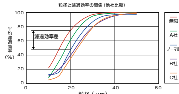
【粒径と通過効率の関係グラフ】上のグラフはスラッジ(異物)の粒径と通過効率の関係を示したグラフです。通過効率がノーマル比で最大36%向上している事が認められます。
