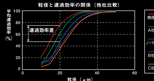
グラフは、スラッジ(異物)の粒徑と濾過効率の関係を示したものです。濾過効率がノーマル比で最大36%向上していることが認められます。
