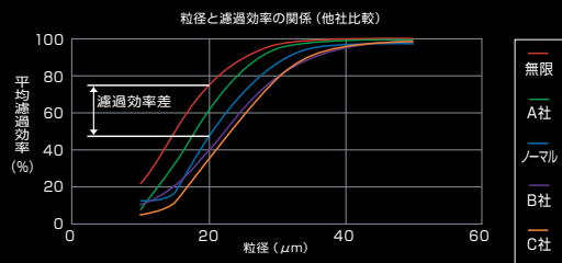
【粒径と濾過効率の関係 グラフ】 上のグラフはスラッジ（異物）の粒径と濾過効率の関係を示したグラフです。濾過効率がノーマル比で最大36%向上している事が認められます。
