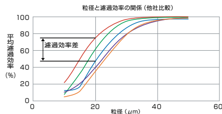
【粒径と濾過効率の関係 グラフ】
